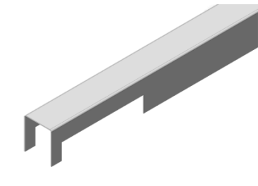
Distansstag, anpassas efter kassett
