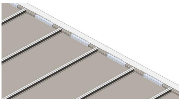
B. Systemöversikt, ovansida – detalj panel med panelclips kopplad mot skuggprofil
